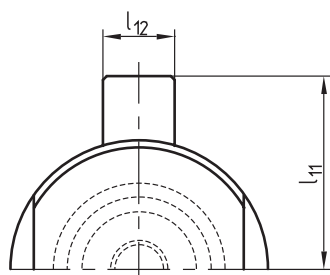
Ansicht/View/Vue „X“
